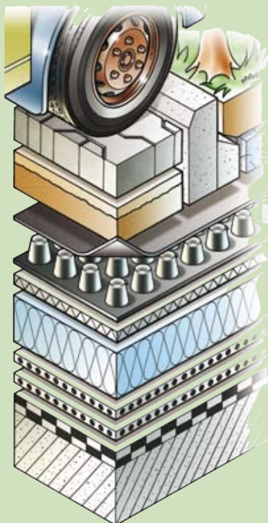
Opbouw omgekeerd-dak met berijdbare verharding
