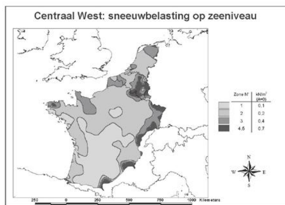
Figuur C.7 – Centraal West: sneeuwbelasting op zeeniveau
